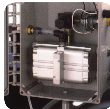
Rotorenhet för tvilling alt. Singelhjul
